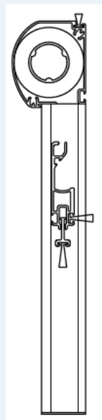
Doorsnede profiel
