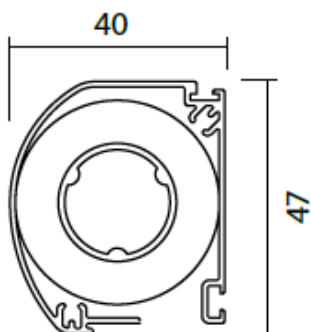
Zijaanzicht
