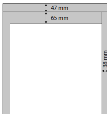
Doorsnede profiel
