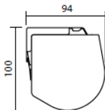
Zijaanzicht cassette
