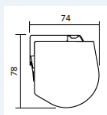
Zij-aanzicht cassette
