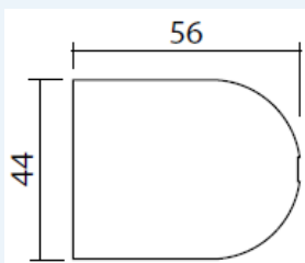
Zij-aanzicht beugel
