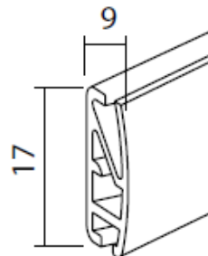
Onderlat
