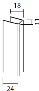
Zijstrips (U-profiel)
